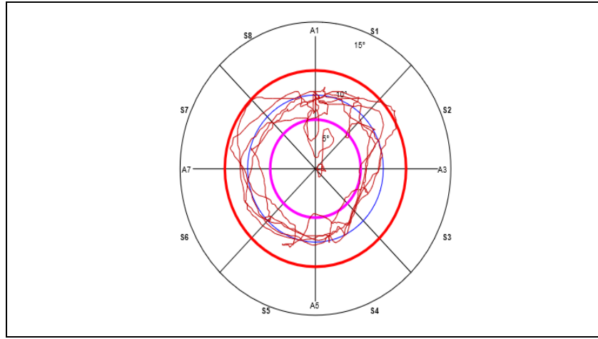
Şekil 10. Sporçunun test esnasında dire içerisinde izlediđi yol
