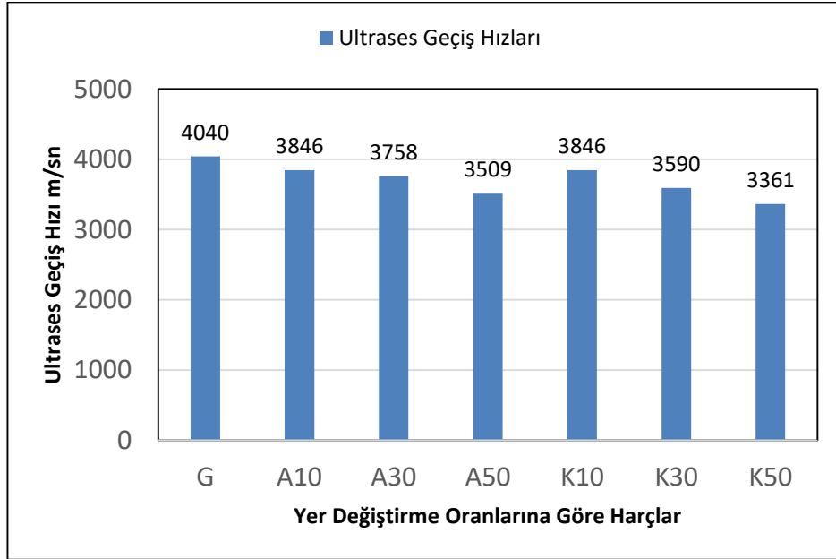
Őekil 5.7 Har numunelerinin ultrases geiř hızı
