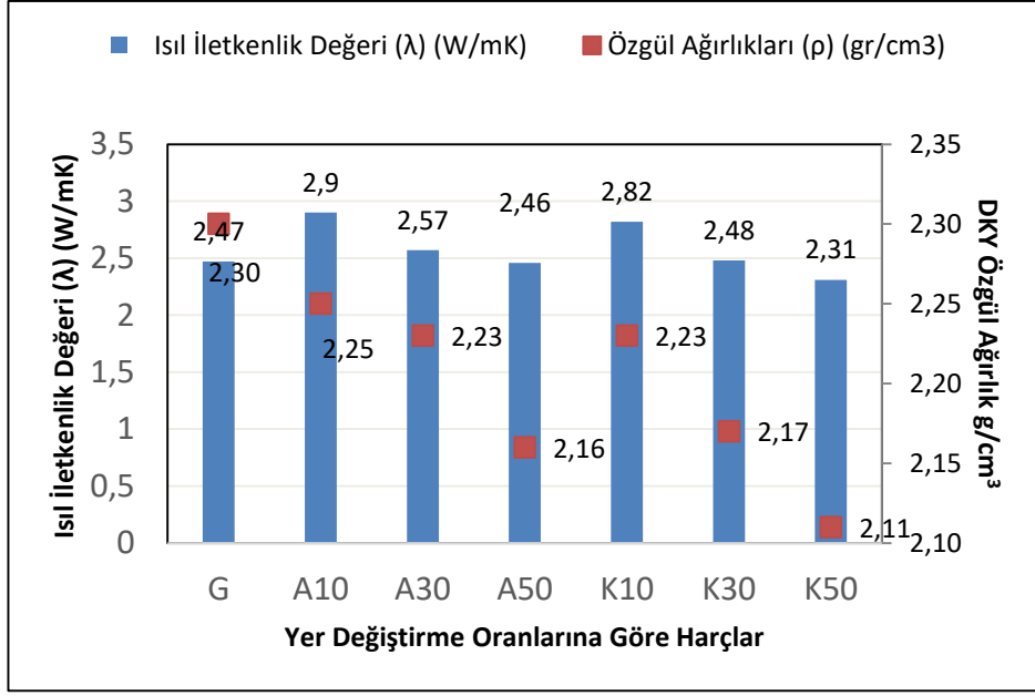
Şekil 5.10 Harç numunelerinin ısı iletkenlik-özgül ağırlığı
