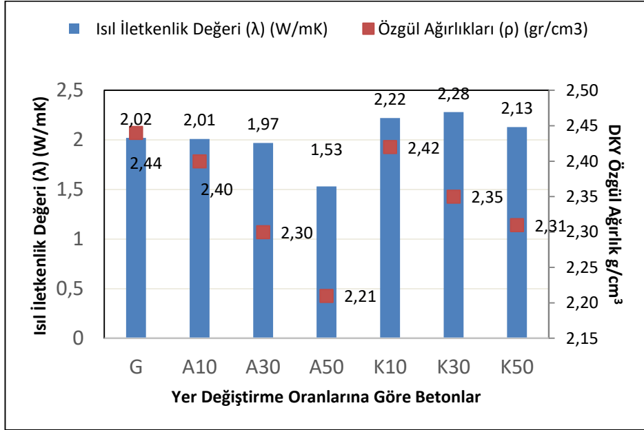
Şekil 5.11 Beton numunelerinin ısı iletkenlik-özgül ağırlığı
