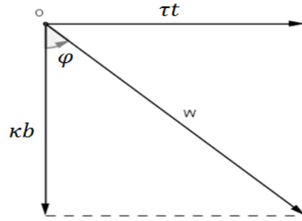
Şekil 3.1.1. Darboux vektörü
