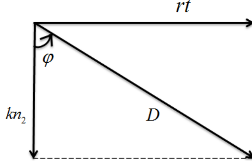
Şekil 3.2.2. Kuaterniyonik Darboux vektörü
