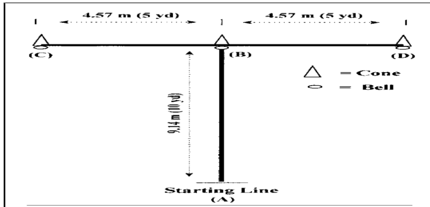
Şekil 2.4. T Testi (Pauole ve ark.)
