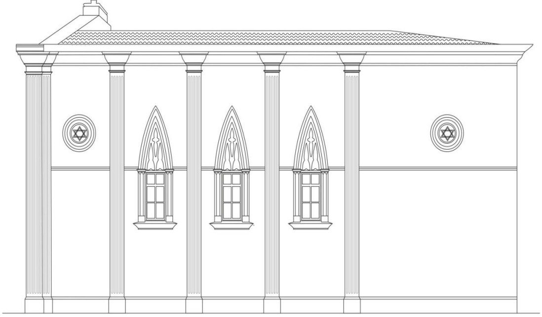
Şekil 14. Giresun Eski Katolik Kilisesi Batı Cephe (Çizim: Semanur Sarımahmutođlu)
