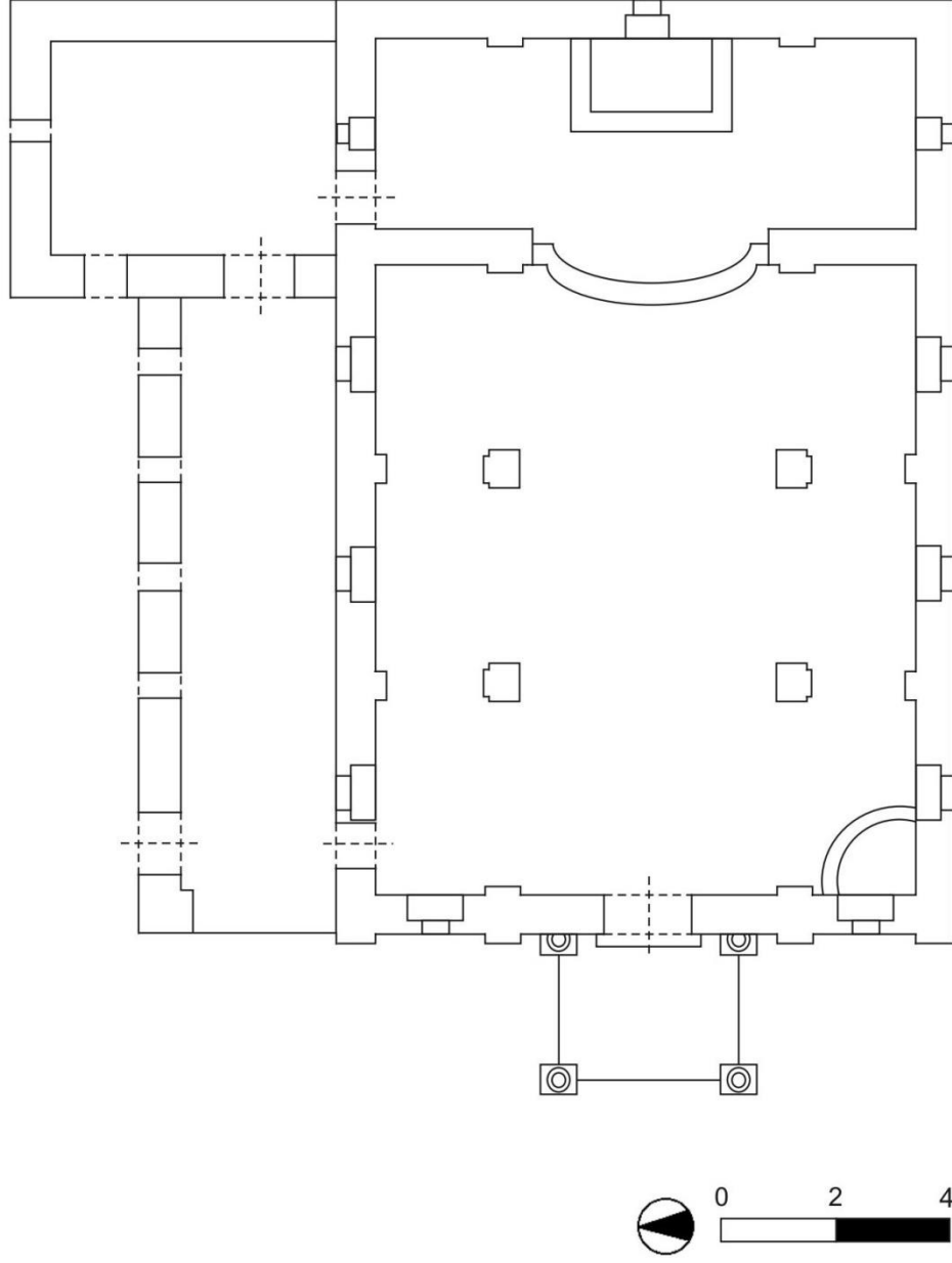
Şekil 2. Trabzon Santa Maria Katolik Kilisesi Planı (Zenbilci, 2019, 61, İşlenerek)
