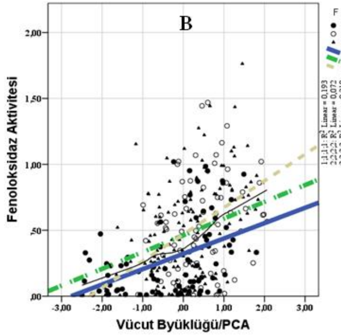
Şekil.4.11. Vücut Büyüklüğünün, Litik Aktivite (A), Fenolksidaz Aktivitesin (B) ile Olan İlişkileri
