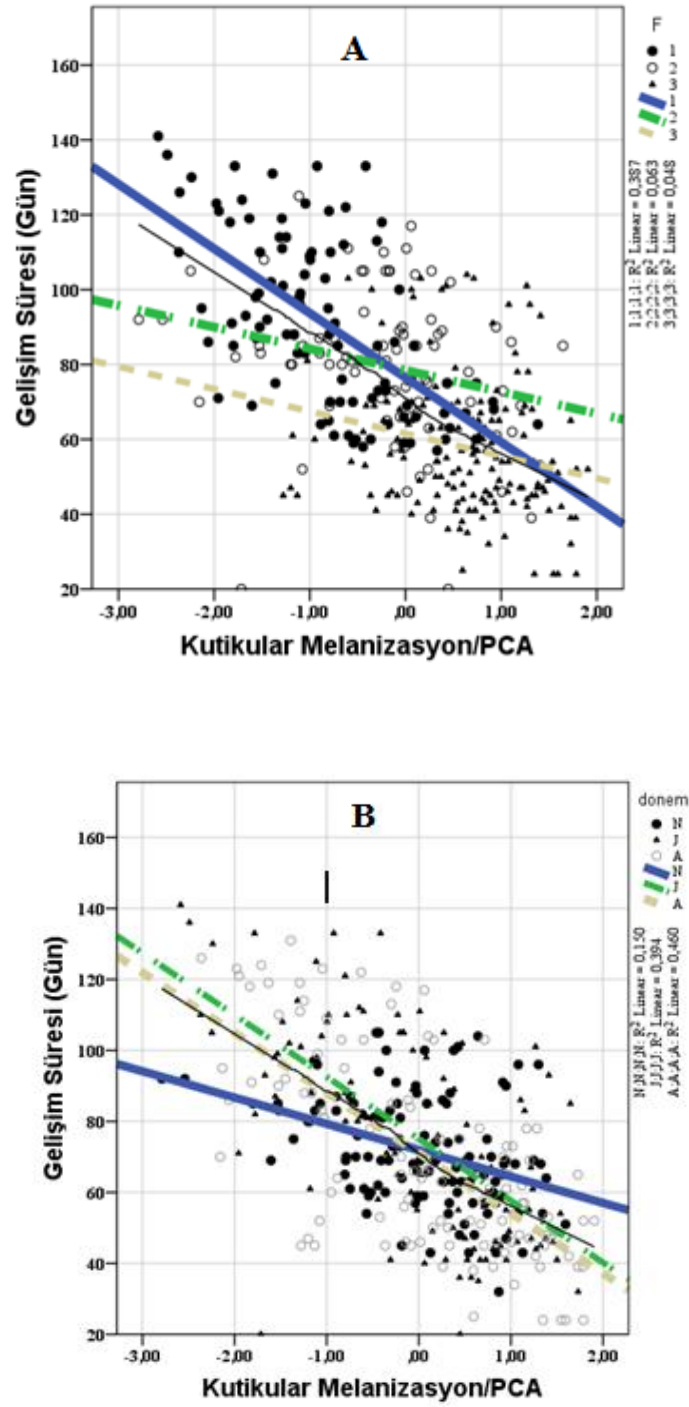
Şekil.4.12. Kutikular Melanizasyonun Gelişim Süresi ile Gelişim Dönemlerine Göre Gösterdiği İlişki
