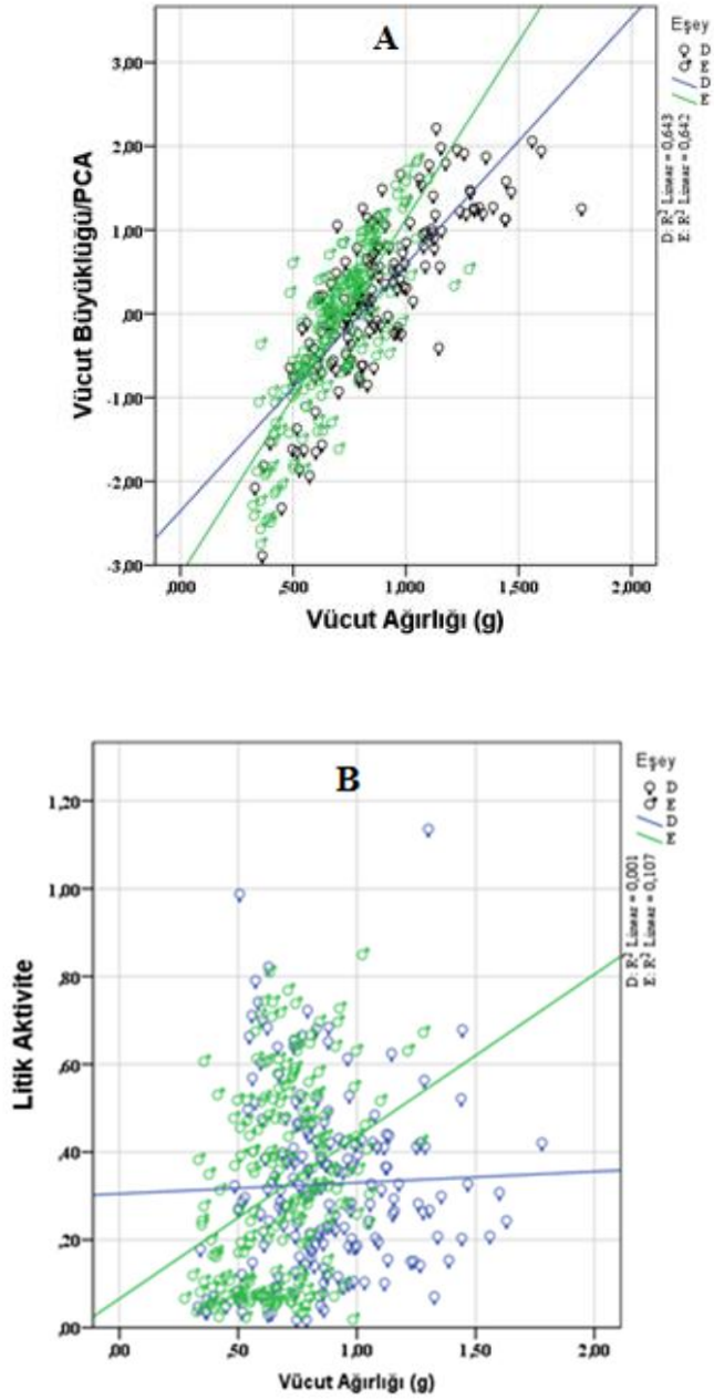
Şekil.4.15. Vücut Ağırlığının, Vücut Büyüklüğü/PCA (A) Ve Litik Aktivite (B) Verileriyle Eşeye Göre Olan İlişkisi
