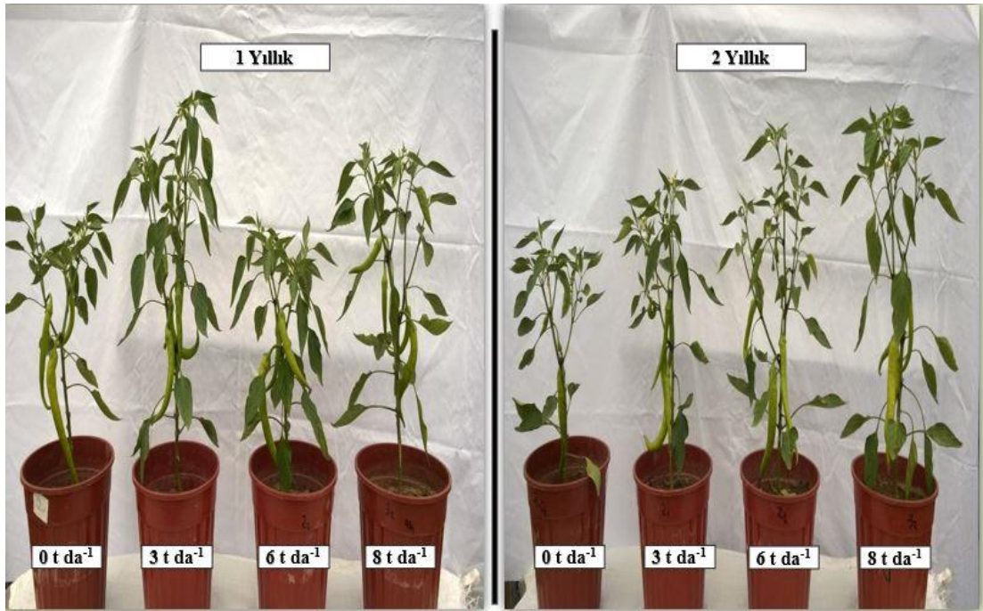
Şekil 4.7. Fındık züruf uygulamalarının bitki boyu üzerine etkisi
