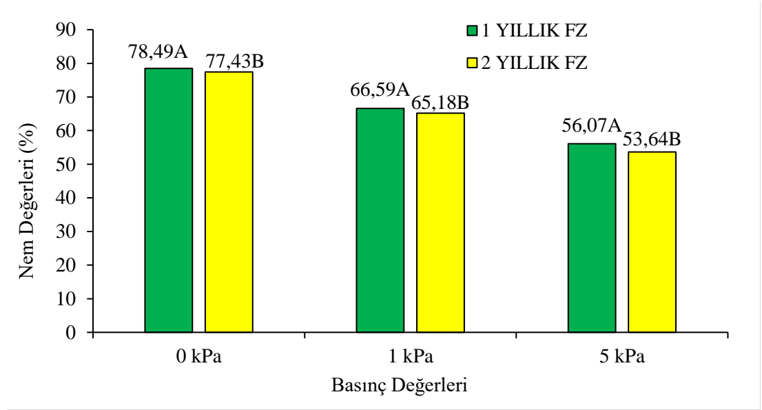
Şekil 4.1. Farklı ayrışma süresinin toprak nem içeriklerine etkisi
