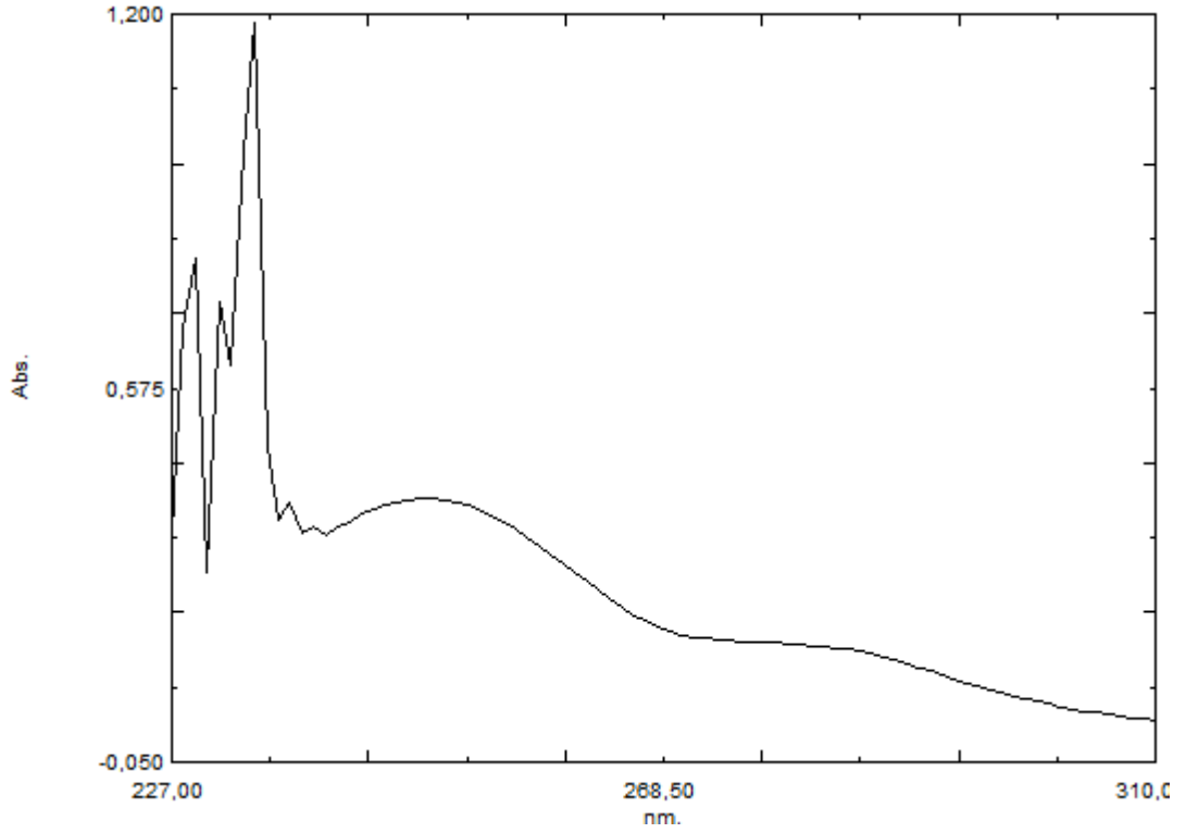
Şekil 4.15. Bileşik 1 'in UV-Vis. spektrumu (CHCl 3 )
