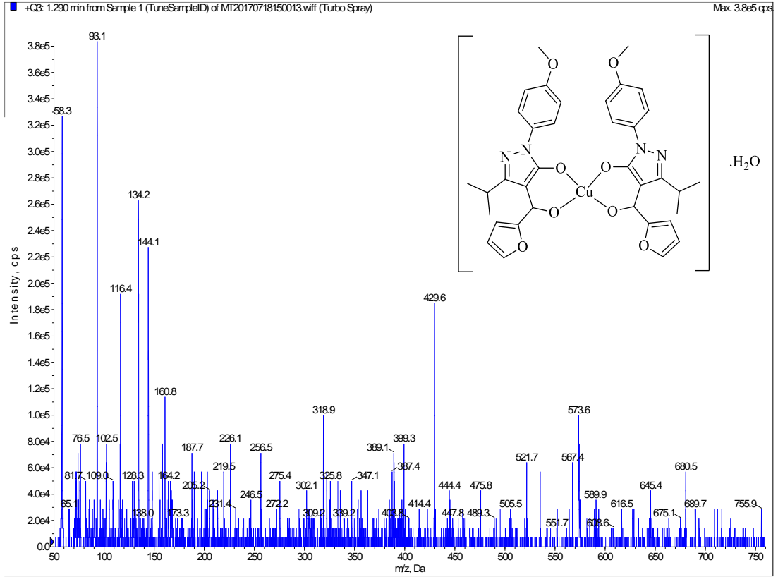
Şekil 4.45. Bileşik 5 'in ESI (+) -MS spektrumu
