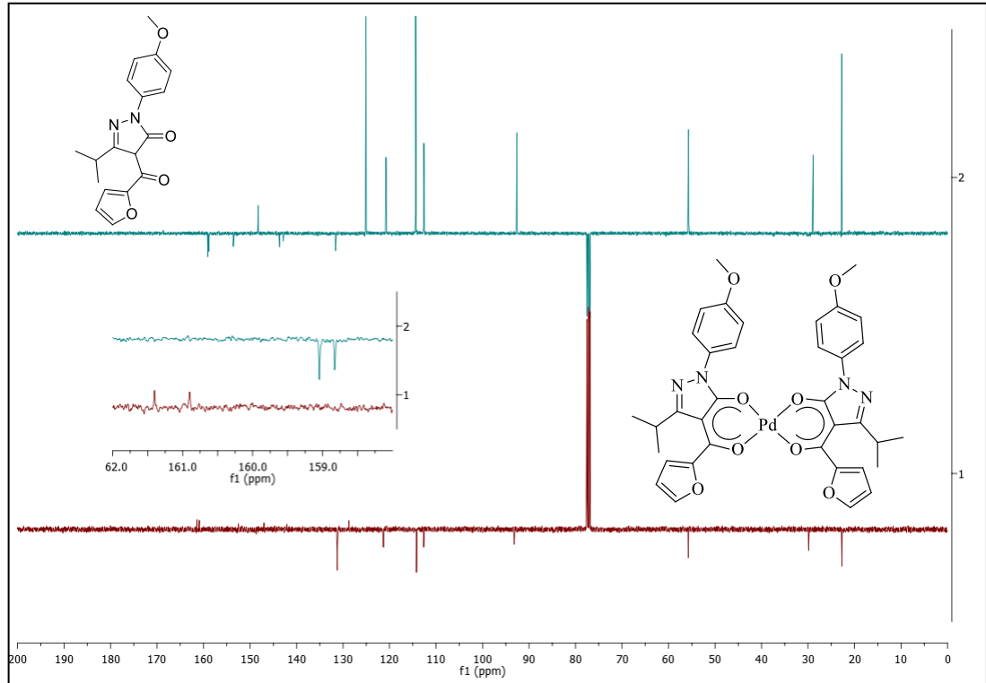
Şekil 5.6. Bileşik 3 ve Bileşik 7 'nin karşılaştırmalı 13 C/APT spektrumları
