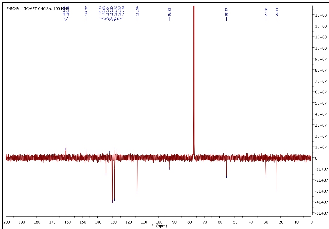
Şekil 4.52. Bileşik 6 'nin ^{13}\text{C} /APT spektrumu ( \text{CHCl}_3\text{-d} )
