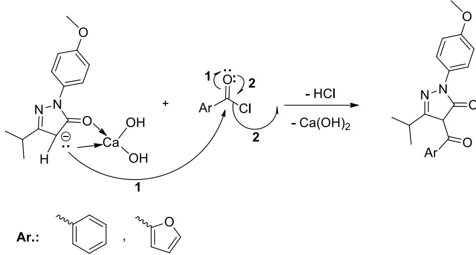
Şekil 5.2. ‘4-Aroil-3-izopropil-1-(4-metoksifenil)-1H-pirazol-5(4H)-on’ bileşiği sentezine ait önerilen reaksiyon mekanizması
