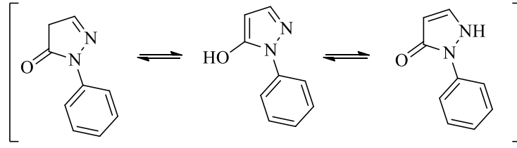
Şekil 1.1. 5-Fenil pirazolonun enol-keto tautomerisi
