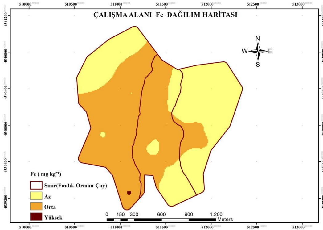
Şekil 4.15 Çalışma Alanı Fe Dağılım Haritası
